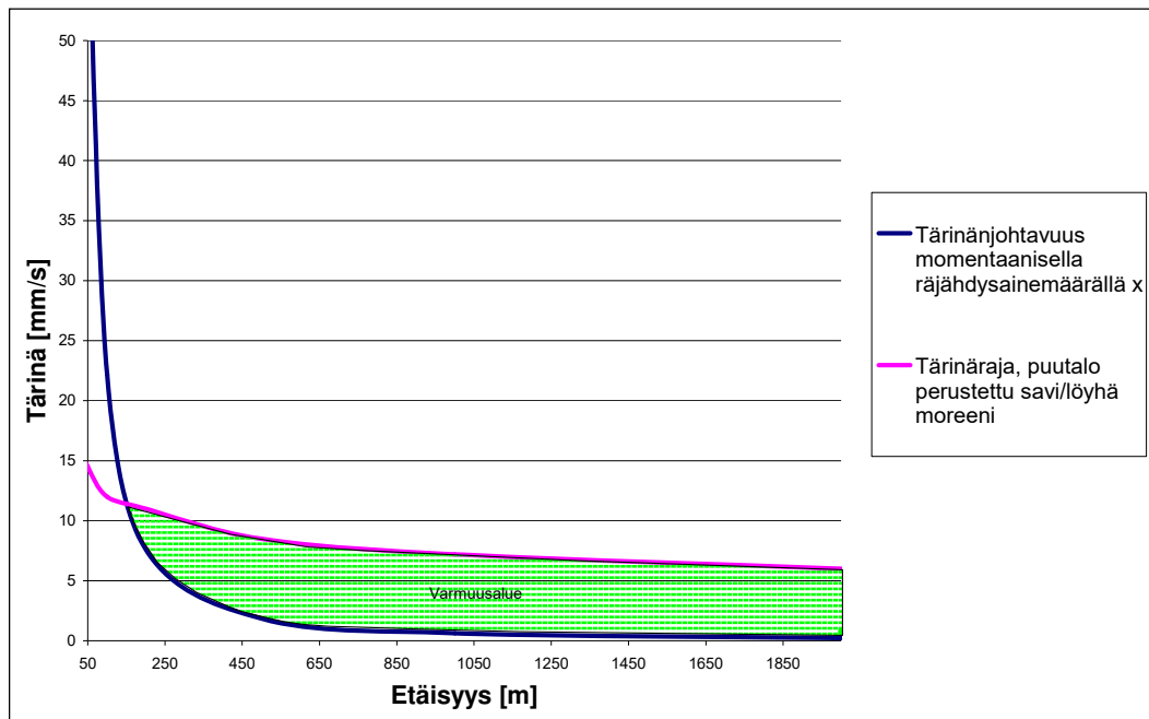
Kuva 5.82. Hankealueen määräysten mukainen värinärakia ja nykyisten värähtyksen aiheuttamat värinät etäisyyden suhteen.
