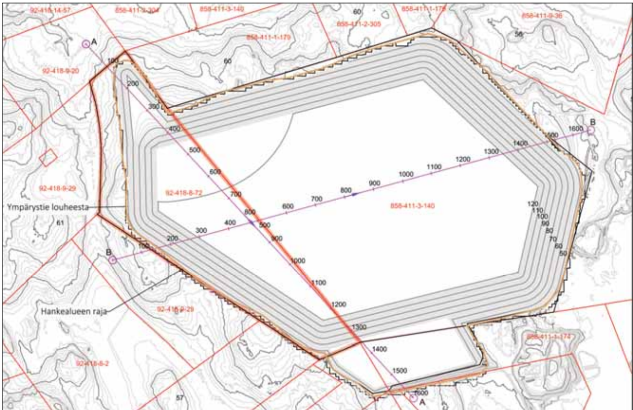
Kuva 1.4. Hankesuunnitelma. Kuvassa on esitetty korkein täyttömäkivaihtoehto, jossa mäen huippu on tasolla +120. Kulku hankealueelle on Tuusulan puolelta Senkkerin nykyiseltä kivasemalta. Bild 1.4. Projektplan. På bilden visas det högsta alternativet för fyllnadsbacken där backens topp ligger på nivån +120. Förbindelse till projektområdet från Tusbysidan går från Senkkeris nuvarande krosstation.
