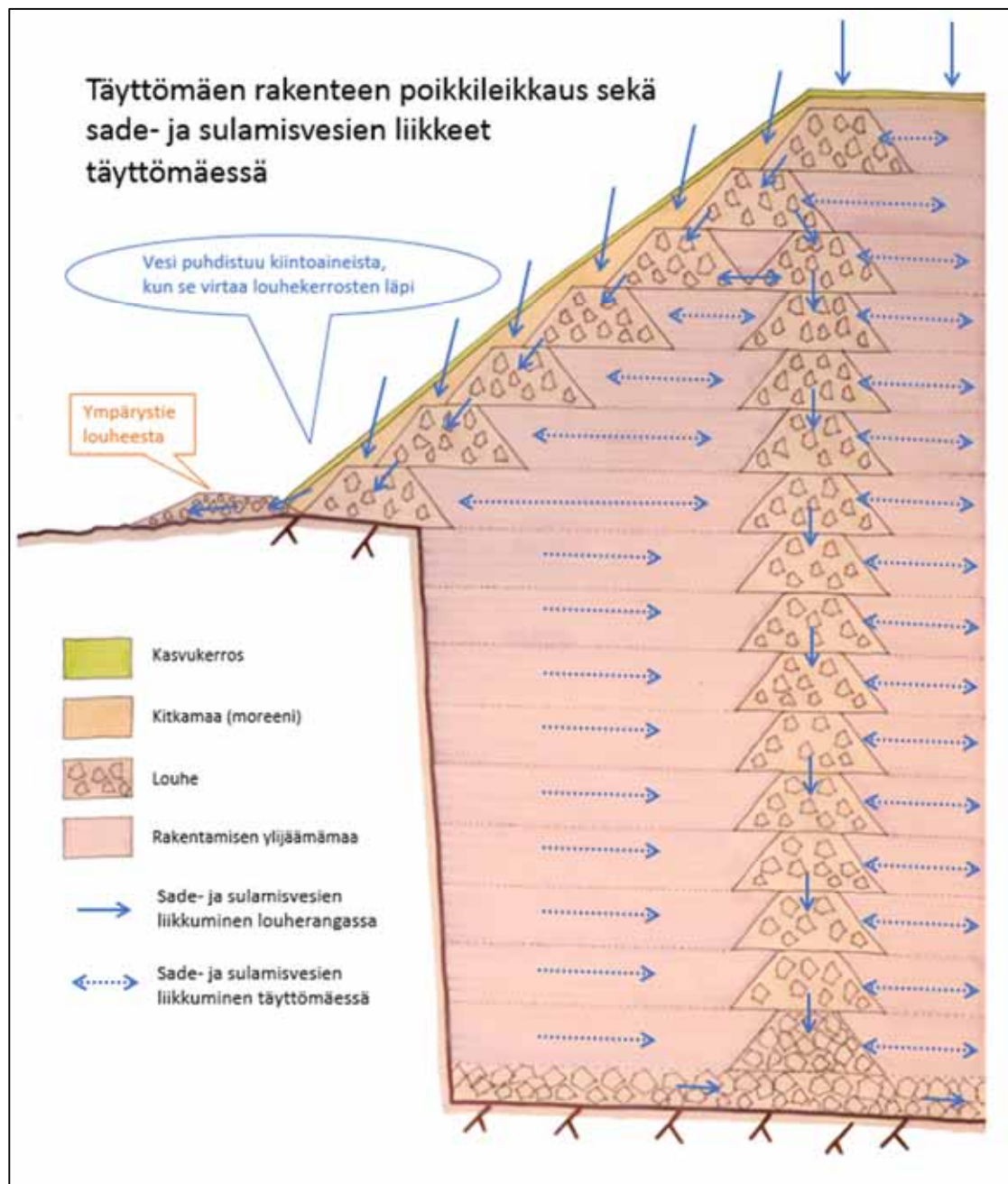
Kuva 1.8. Havainnollistava kuva vesien liikkeistä täyttömaässä. Bild 1.8. En illustrativ bild av vattenrörelser på fyllningsbacken.
