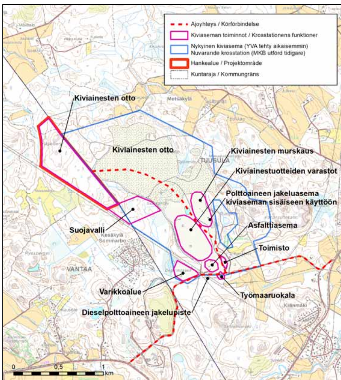
Kuva 1.2. Hankealueen ja viereisen kiviaseman toiminnot.
