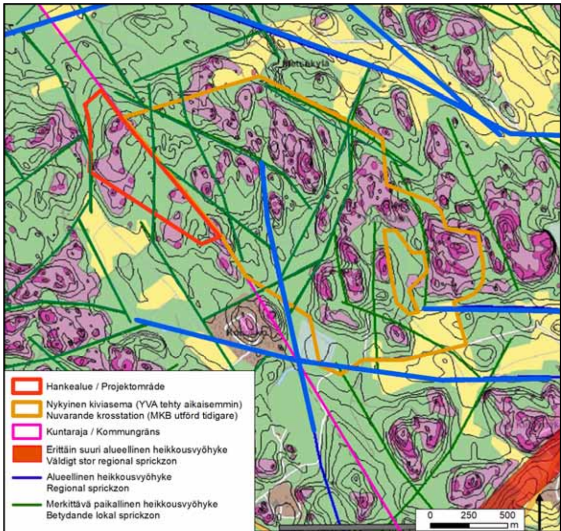
Kuva 5.3. Kallion rakennettavuuskartta. Bild 5.3. Karta över bergets byggbarhet.
